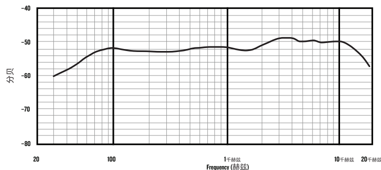
频率响应图
